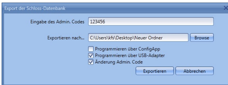
Afb. 134: Wijzigen van de admin. code
