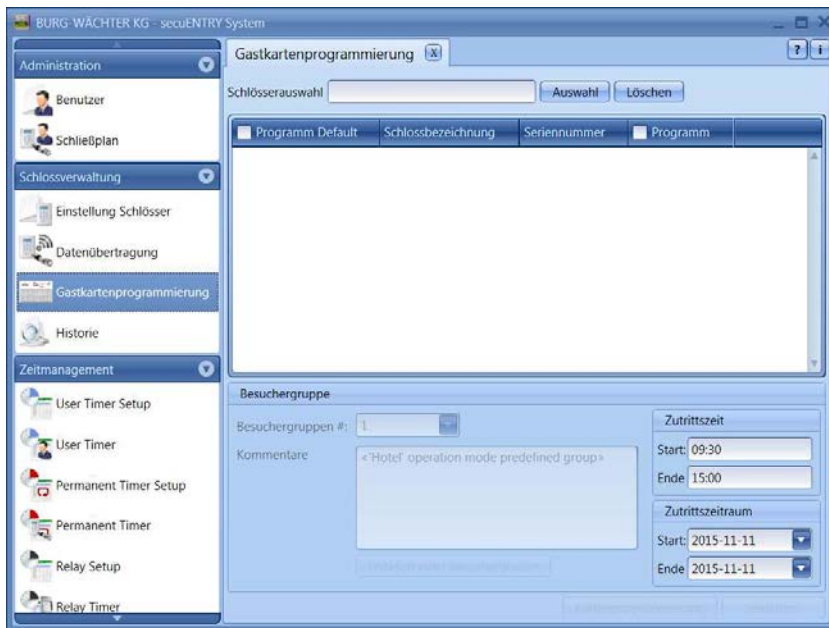
Afb. 156: Gastkaartenprogrammering ENTRY System +
